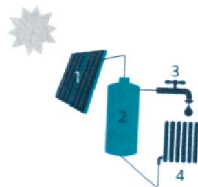
1. Zonnecollector | 2. Opslagvat zonneboiler | 3. Sanitair warm water | 4. Afgifta-element voor ruimteverwarming (optioneel)
